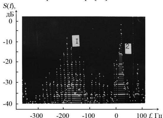
Рис. 7. Текущий спектр эхо-сигналов от вертолета типа Ка-26 на волне 35 см: 1 – спектр эхо-сигналов от вертолета; 2 – спектр эхо-сигналов от моря
