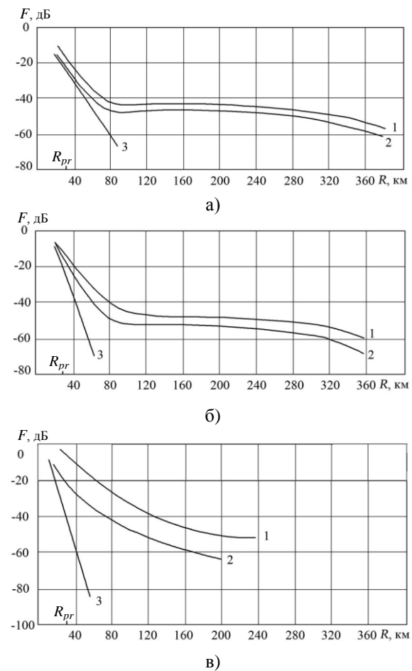
Рис. 1. Множители ослабления поля на открытых морских трассах: а) – \lambda=35 см; б) – \lambda=10 см; в) – \lambda=3 см; 1 – южные широты Атлантики; 2 – северные широты Атлантики; 3 – расчет по дифракционным формулам
