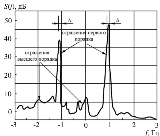
Рис. 5. Усредненный спектр на волне 6,4 МГц, T_{ус} = 100 с, \Delta – смещение спектра за счет поверхностных течений
