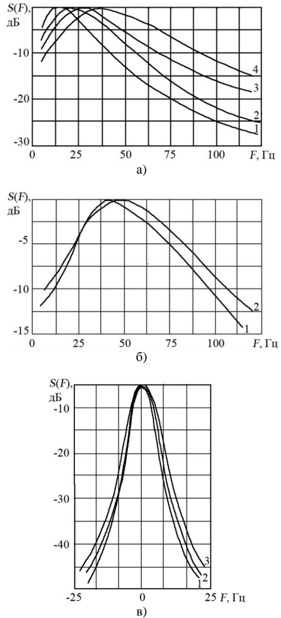
Рис. 2. Влияние силы волнения на форму спектров рассеянных сигналов. Поляризация излучения вертикальная: а) – \lambda=10 см; H_w=0,6 м; 0,6-1,2 м; 1,2-1,8 м; 1,8-4 м (кривые 1-4); б) – \lambda=30 см; H_w=0,8 -1 м; 1-1,2 м (кривые 1, 2); в) – \lambda=30 см; H_w=1,5 , 2,1 и 3,25 м (кривые 1-3); г) – \lambda=2 м; H_w=0,3 -1 м; 1-2 м (кривые 1, 2)
