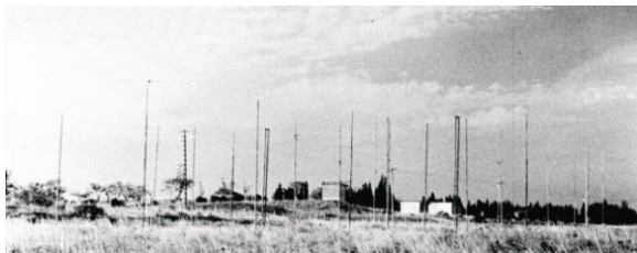
Рис. 4. Антенное поле 3-х частотного дкм локатора поверхностной волны
