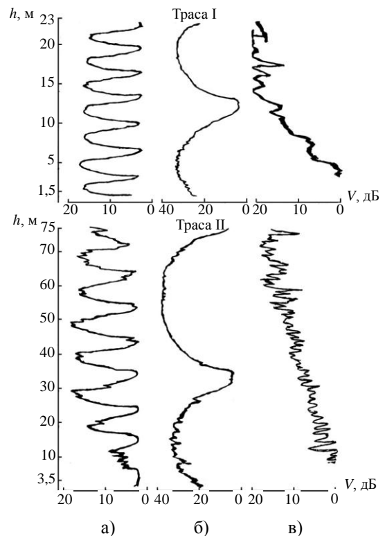
Рис. 6. Примеры записи высотной структуры поля на I и II трассах. Трасса I – R = 8 км, трасса II – R = 22 км: а) – \lambda = 8 мм; б) – \lambda = 4 см; в) – \lambda = 35 см
